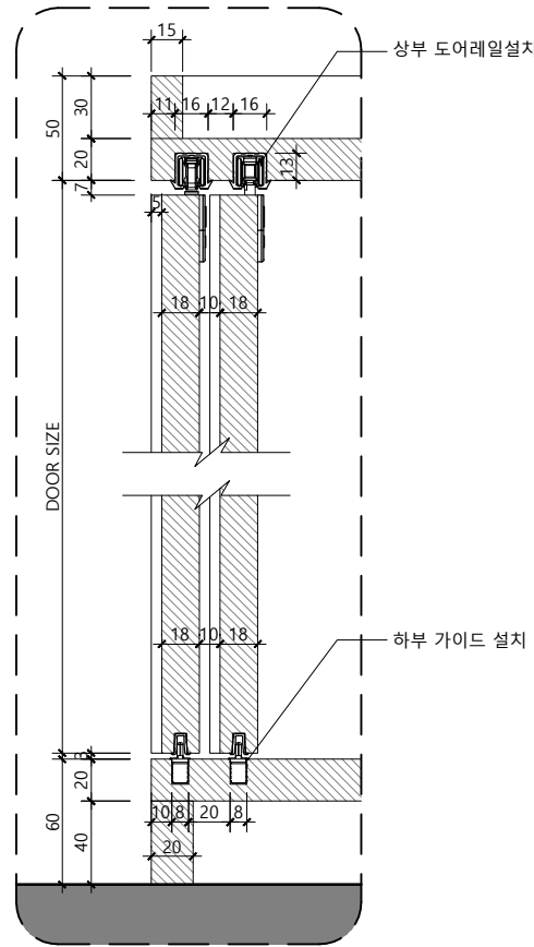
상부 도어레일
